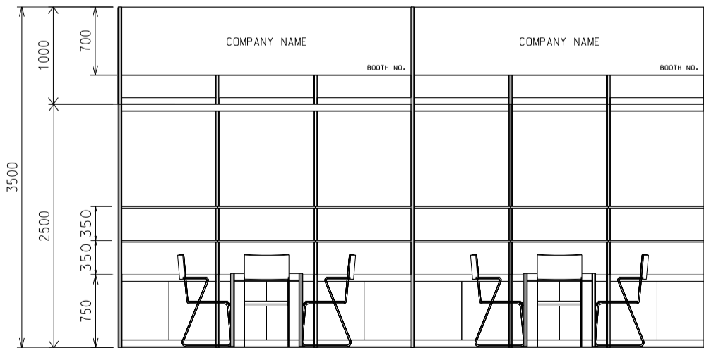
ELEVATION 6M(W) X 3M(D) X 3.5M(H)
